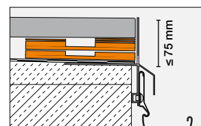
Randprofil Schlüter®-BARA-RKLT
