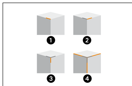
Ordre des étapes de travail pour la pose d'angles à 3 côtés
